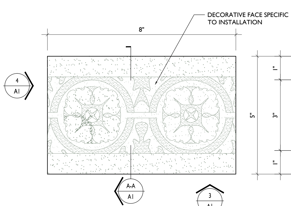
1 FRONT A1 Scale: 6" = 1'-0"
